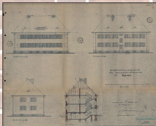
Plany budynku niemieckiego Urzędu Celnego w Dębowej Łące (Geyersdorf), 1937 r. [APZG, Komisariat Obwodowy Wschodnia-Północ, sygn. 15]
